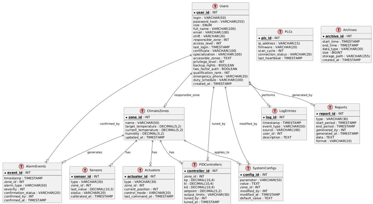
Рисунок 1 - ER-диаграмма
